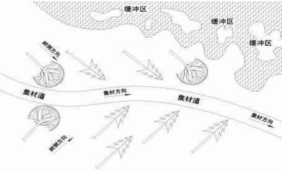
图 1 采伐带树木倒向图
