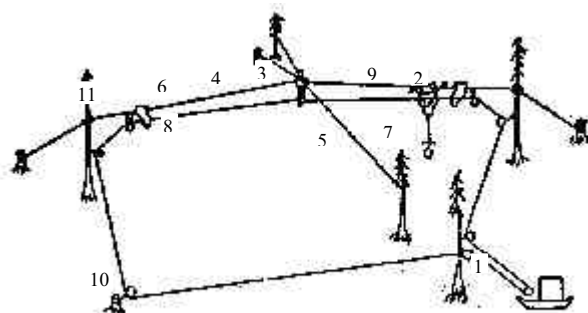
图 5 索道的组成
