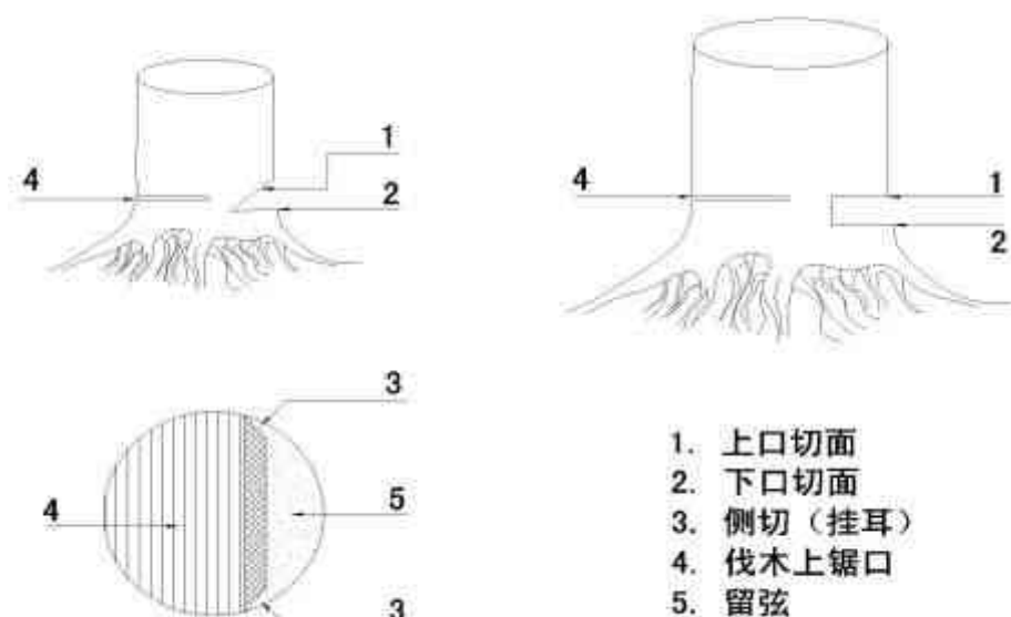
图 3 采伐示意图
